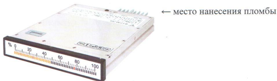
Рисунок 1 – Амперметры и вольтметры узкопрофильные Ф1730
