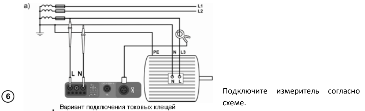
Вариант подключения токовых клещей
