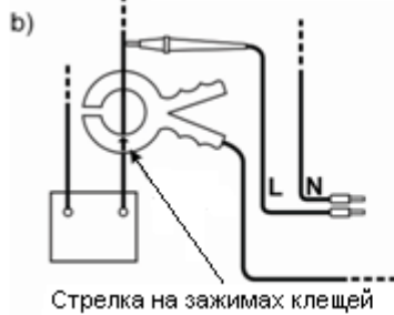
Вариант подключения токовых клещей
