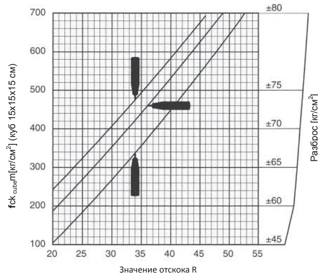
Рис. 2.8 Тип L/LR: кривые перевода, построенные на основании средней прочности на сжатие куба и значении отскока R.
