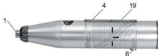
Рис. 2.4 Считывание результатов проведенного испытания по шкале (19) молотка
