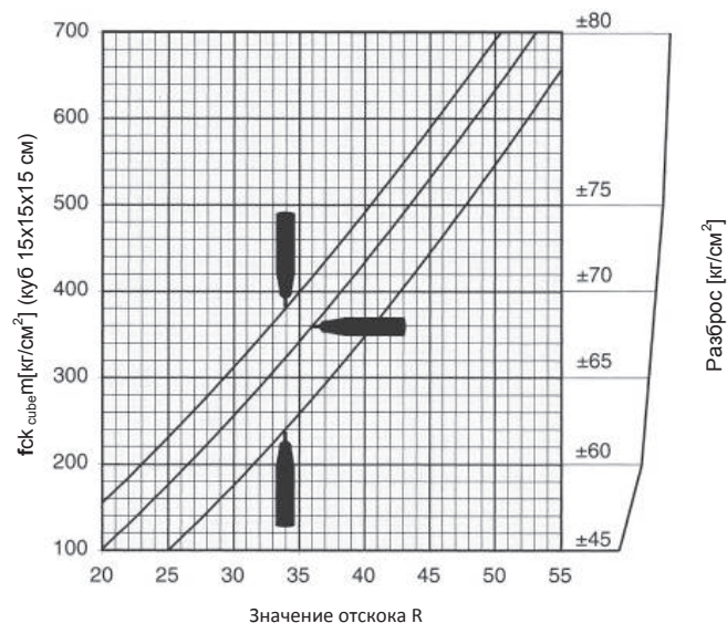
Рис. 2.7 Тип N/NR: кривые перевода, построенные на основании средней прочности на сжатие куба и значении отскока R.
