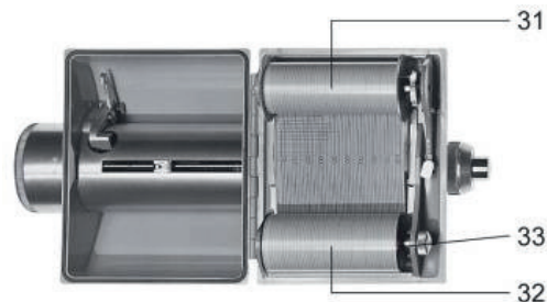
Рис. 3.2. Заправка нового рулона бумажной ленты
