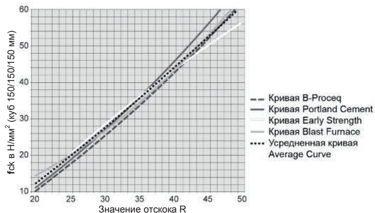
Рис.2.7 Четыре кривые J и кривая Proceq-B
