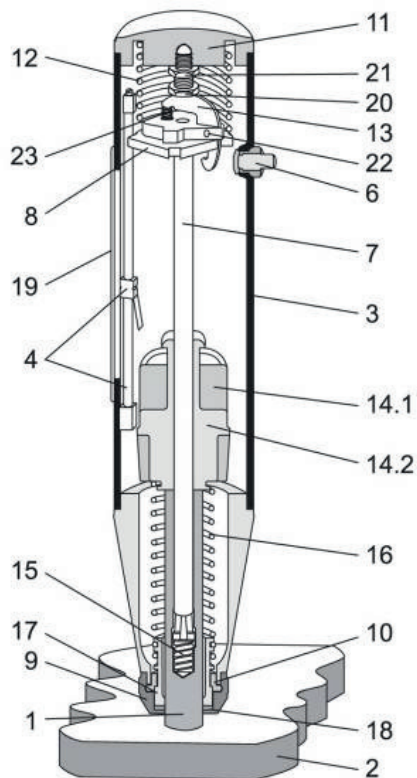
Рис. 3.3 Продольный разрез молотка для контроля бетона
