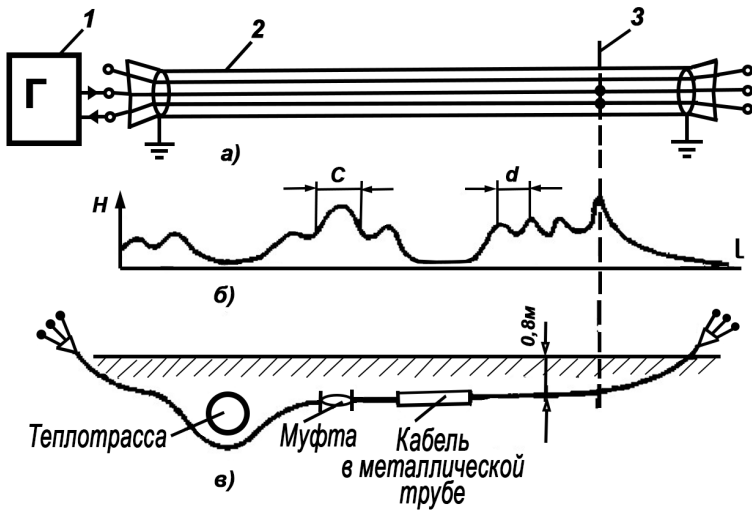
Рис.5.10 КЗ-междуфазное
