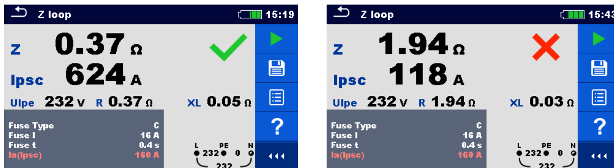
Рисунок 7.30: Пример результатов измерения полного сопротивления контура.
