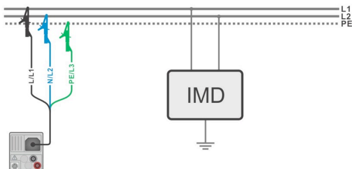
Рисунок 7.68: Измерение наибольшего тока утечки первичного повреждения с 3-проводным кабелем.
