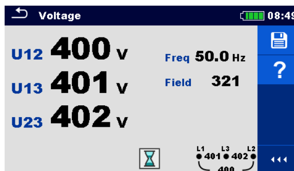
Рисунок 7.5: Пример результатов измерения напряжения в 3-фазной системе.
