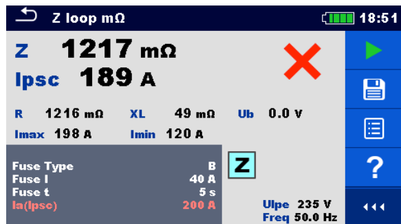
Рисунок 7.37: Пример результатов высокоточного измерения полного сопротивления контура.
