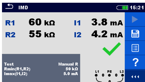
Рисунок 7.73: Пример результатов испытания IMD (устройства контроля изоляции).
