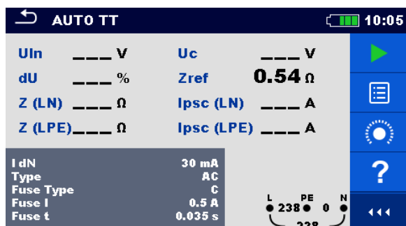
Рисунок 8.5: Примеры с результатов измерения АВТО ТТ.
