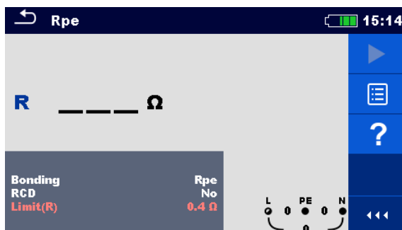
Рисунок 7.74: Меню измерения сопротивления провода защитного заземления.
