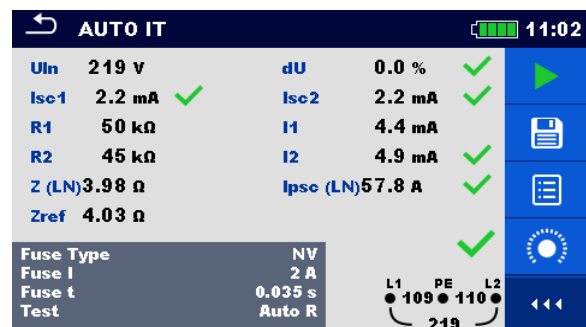
Рисунок 8.14: Примеры с результатов измерения AUTO IT.
