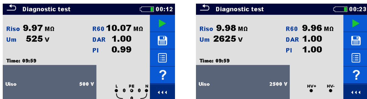
Рисунок 7.13: Примеры результатов диагностического испытания.
