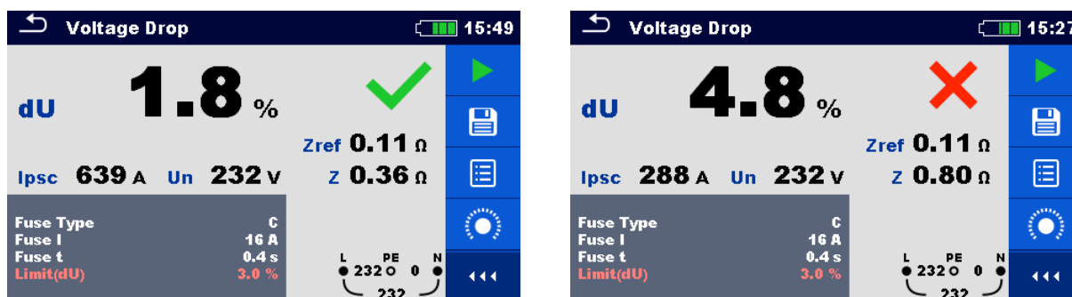
Рисунок 7.47: Пример результатов измерения падения напряжения (шаг 2).
