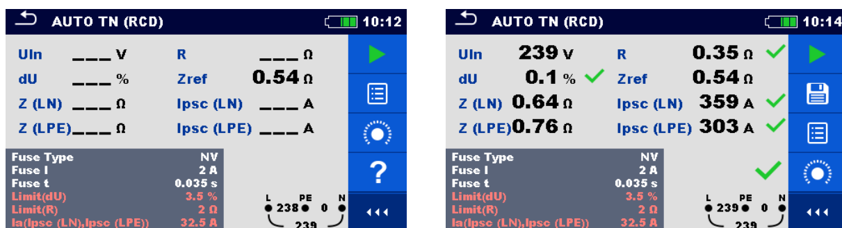
Рисунок 8.8: Примеры результатов измерения АВТО TN (УЗО).
