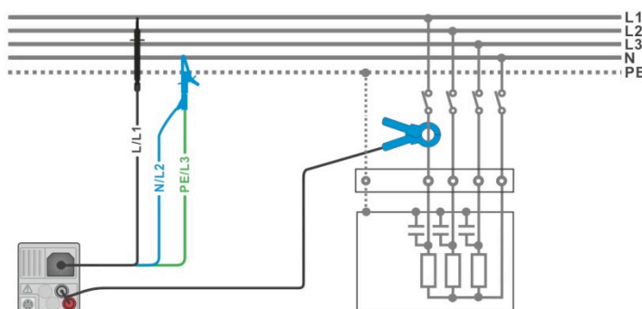
Рисунок 7.59: Измерение мощности.
