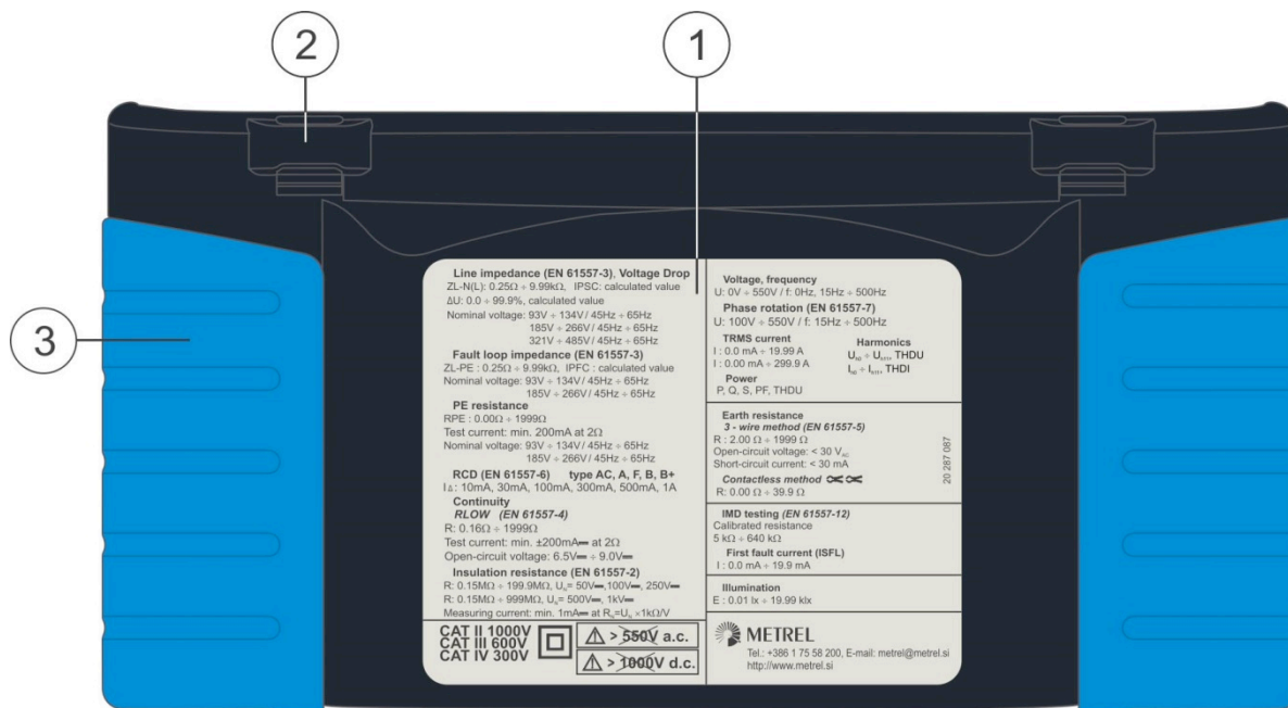
Рисунок 3.5: Вид снизу
