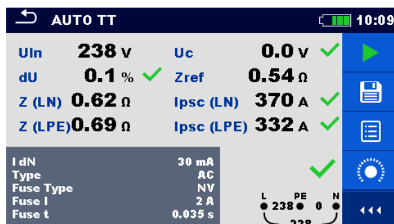
Рисунок 8.5: Примеры с результатов измерения АВТО ТТ.
