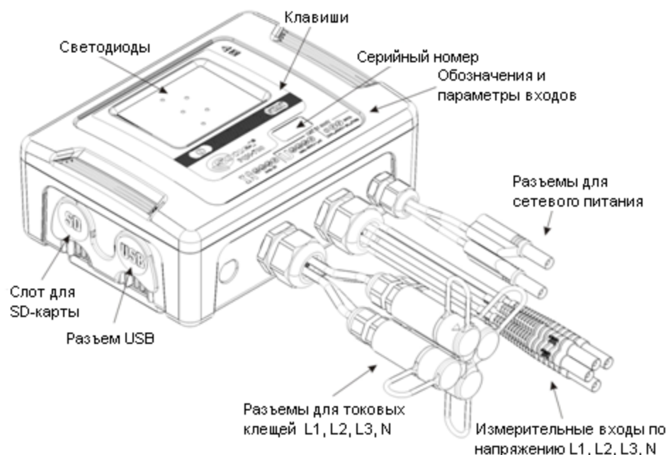
Анализатор качества электрической энергии PQM-700. Общий вид.
