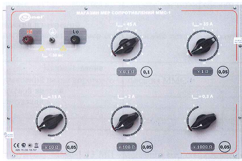
Рисунок 1 – Фотография общего вида магазинов мер сопротивлений петли короткого замыкания ММС-1
