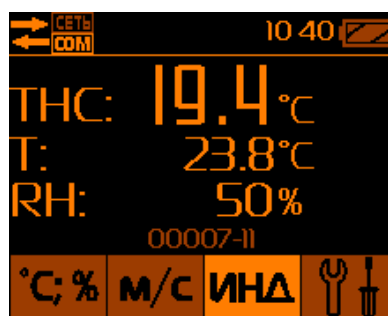
Рис.16 – Определение ТНС-индекса с подключённым датчиком «чёрный шар»
