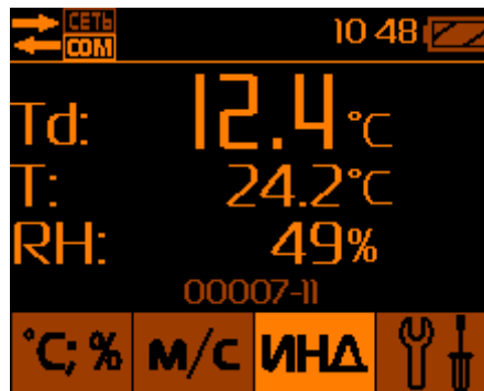
Рис.20 – Режим определения точки росы
