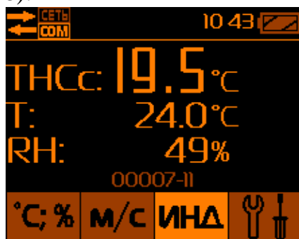
Рис.18 – Определение ТНС-индекса с солнечной нагрузкой
