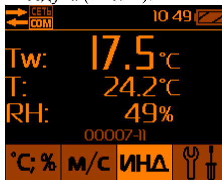
Рис.21 – Режим определения температуры влажного шарика термометра
