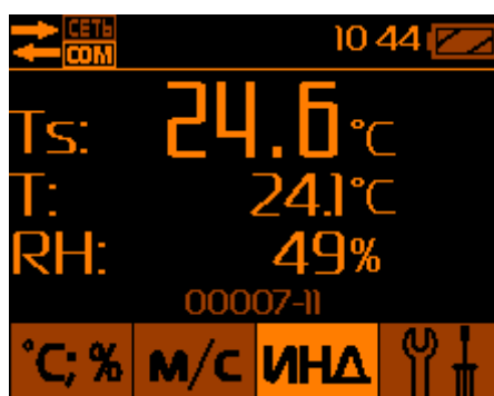
Рис.19 – Режим отображения температуры «чёрного шара»
