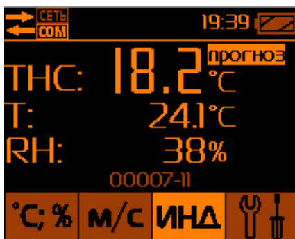
Рис.17 – Прогнозный расчёт ТНС-индекса при отсутствии подключённого «чёрного шара»
