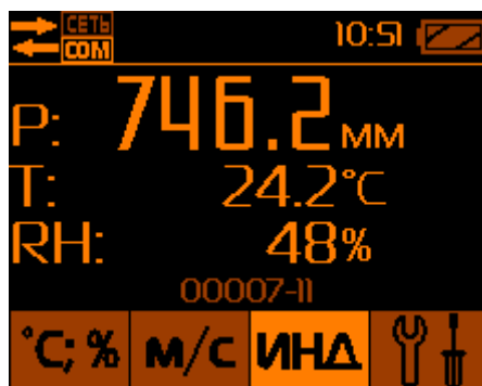
Рис.22 – Режим измерения атмосферного давления.
