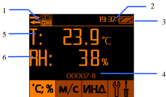
Рис.4 – Измерение температуры и влажности воздуха
