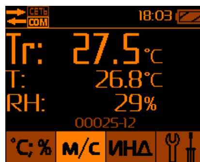
Рис.13 – Измерение радиационной температуры, температуры и влажности.
